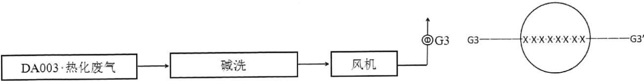
图例：◎—废气检测点位，x—废气测点位置。
